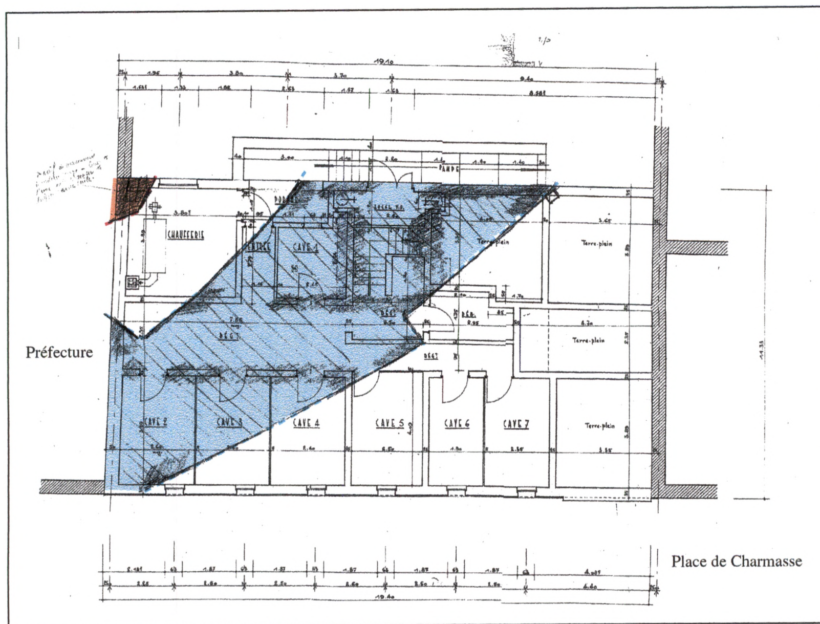
Fig. 3. Plan du sous-sol de la Résidence des Marbres levé par P. Lavadoux (moitié ouest uniquement), annoté par G. Vuillemot en 1963.
