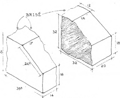
DEUX BLOCS CHANFREINÉS
