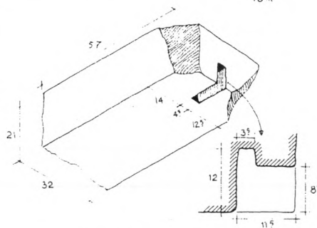
BLOC AYANT UNE MORTAISE » BARDAGE
