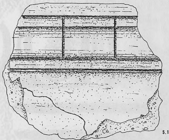
fig.13 : AUTUN. CLINIQUE DU PARC. CORNICHE, TYPE 5. RELEVÉ ET DESSIN : J-F. LEFEVRE. CEPMR-CNRS. 1993.
