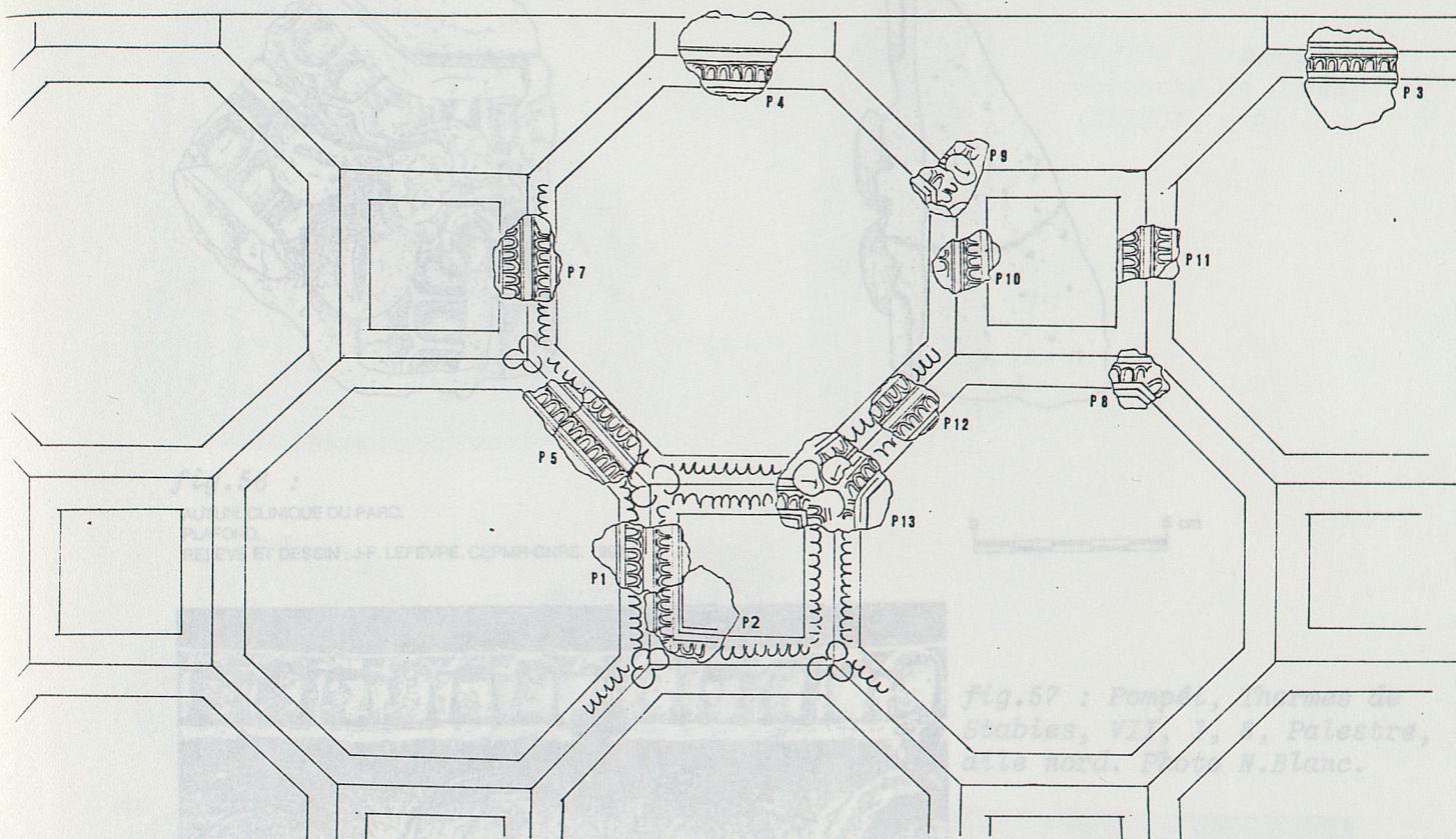
fig.54 : AUTUN, Clinique du Parc, voûte. Dessin et restitution S. Groetembril, CEPMR-CNRS, 1993.
