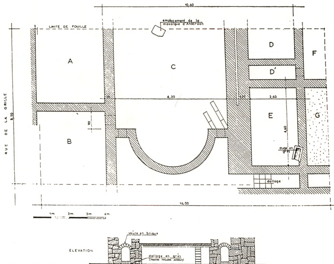
Figure 1. — Plan et élévation de la maison.
