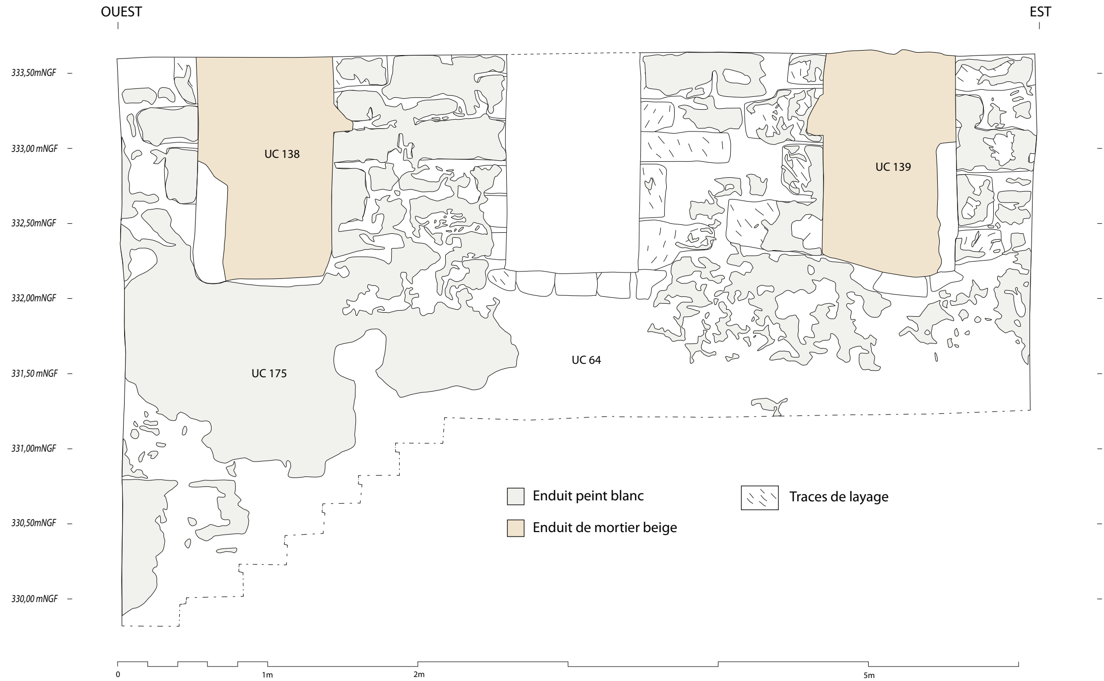
Fig. 71. Organisation des enduits sur le parement intérieur de l'UM 1 (ESP 7). Ech. 1:25. Relevé et DAO: C. Couderc
