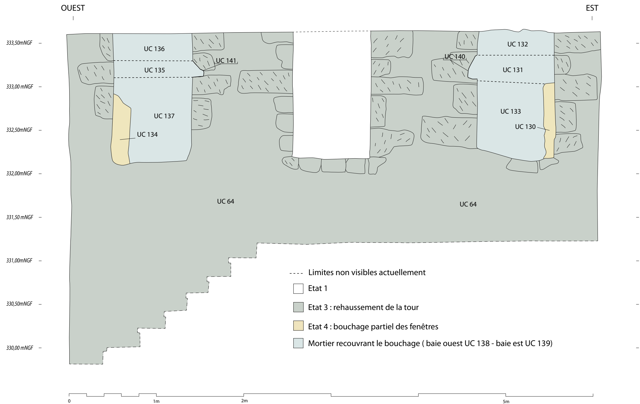
Fig. 67b. Organisation des phases de construction sur le parement intérieur de l'UM 1 (ESP 7). Ech. 1:25. Relevé et DAO: C. Couderc
