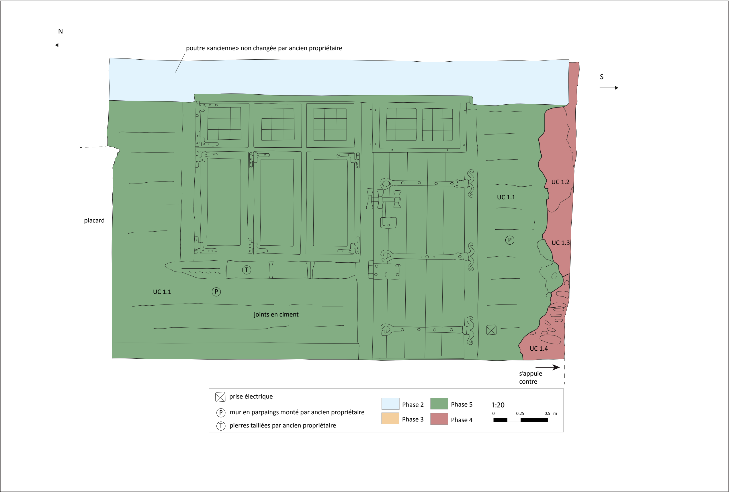
Relevé des phases de construction de l'UM1. Relevé C. Coudrec, DAO A. Tisserand
