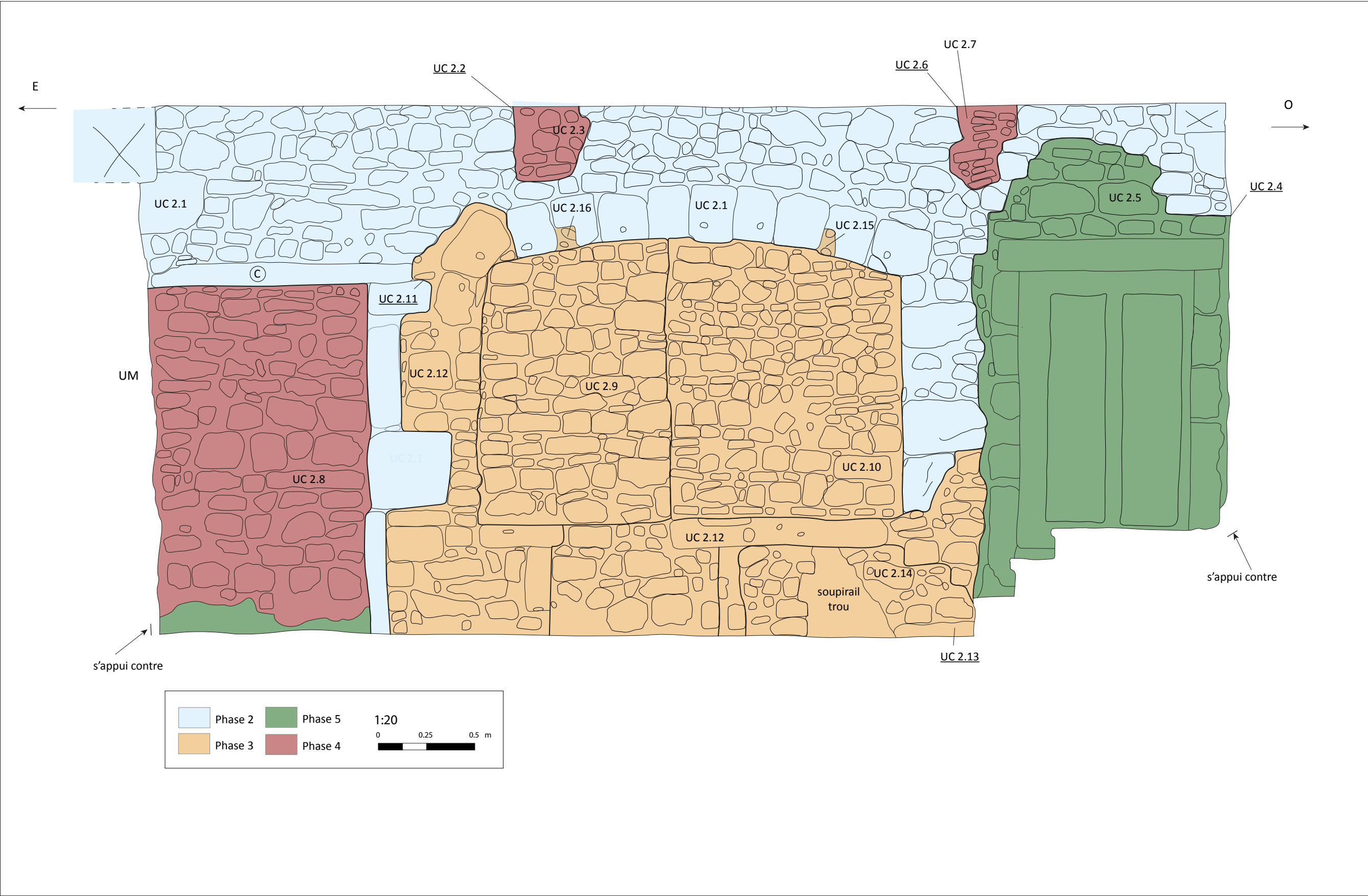
Relevé des phases de construction de l'UM2. Relevé C. Coudrec, DAO A. Tisserand
