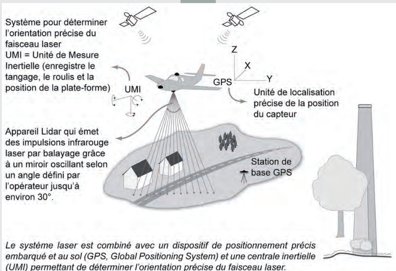
Fig. 1 Principe du système laser aéroporté LIDAR ( Light Détection and Ranging ), (d'après Ž. Kokalj et K. Oštir, in, Rodier et al., 2011)
