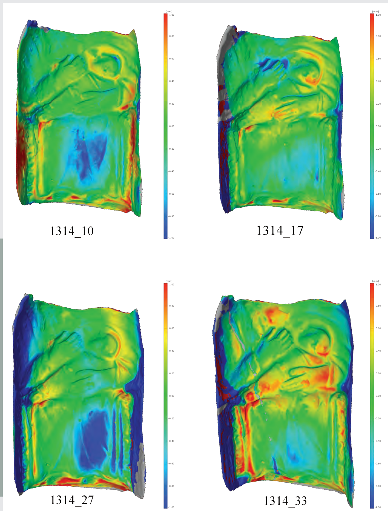
Fig. 7 Résultat de la comparaison de surface des valves de moule sur la valve 1314_9 (Numérisation et traitement L. Androuin).
