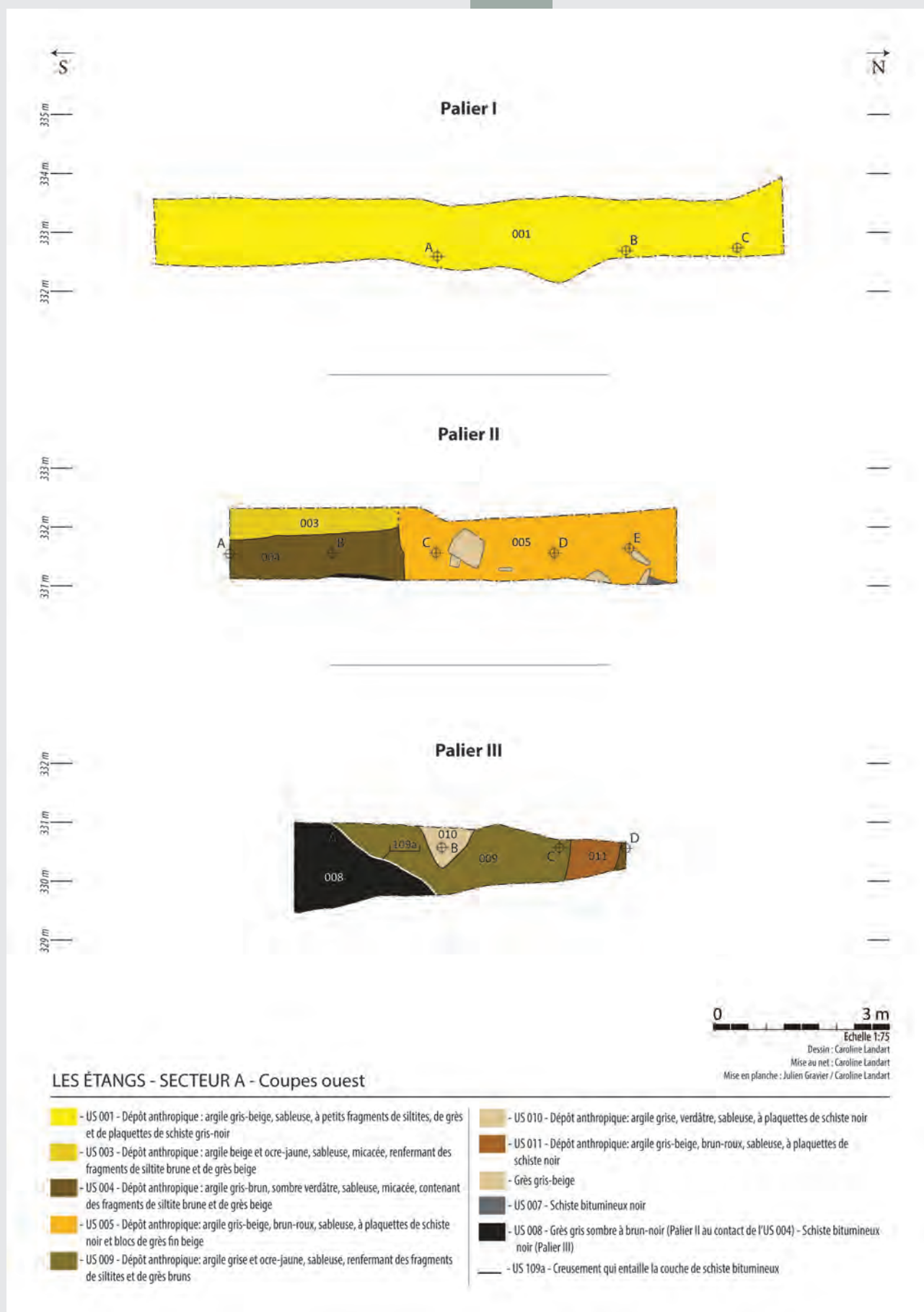
Fig. 6 Coupes ouest adjacentes aux paliers I, II, III dans la dépression. DAO J. Gravier, C. Landart.
