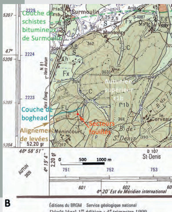
Fig. 2 A : Carte LIDAR de la zone des levées et localisation des deux secteurs fouillés dans le Bois de St-Martin. L'alignement des levées est clairement visible. Source LIDAR Service Archéologique de la ville d'Autun ; DAO B. Ligouis. B : Localisation des secteurs fouillés sur la carte géologique à 1/50 000. Feuille Épinac, n°525, 1999. DAO B. Ligouis.
