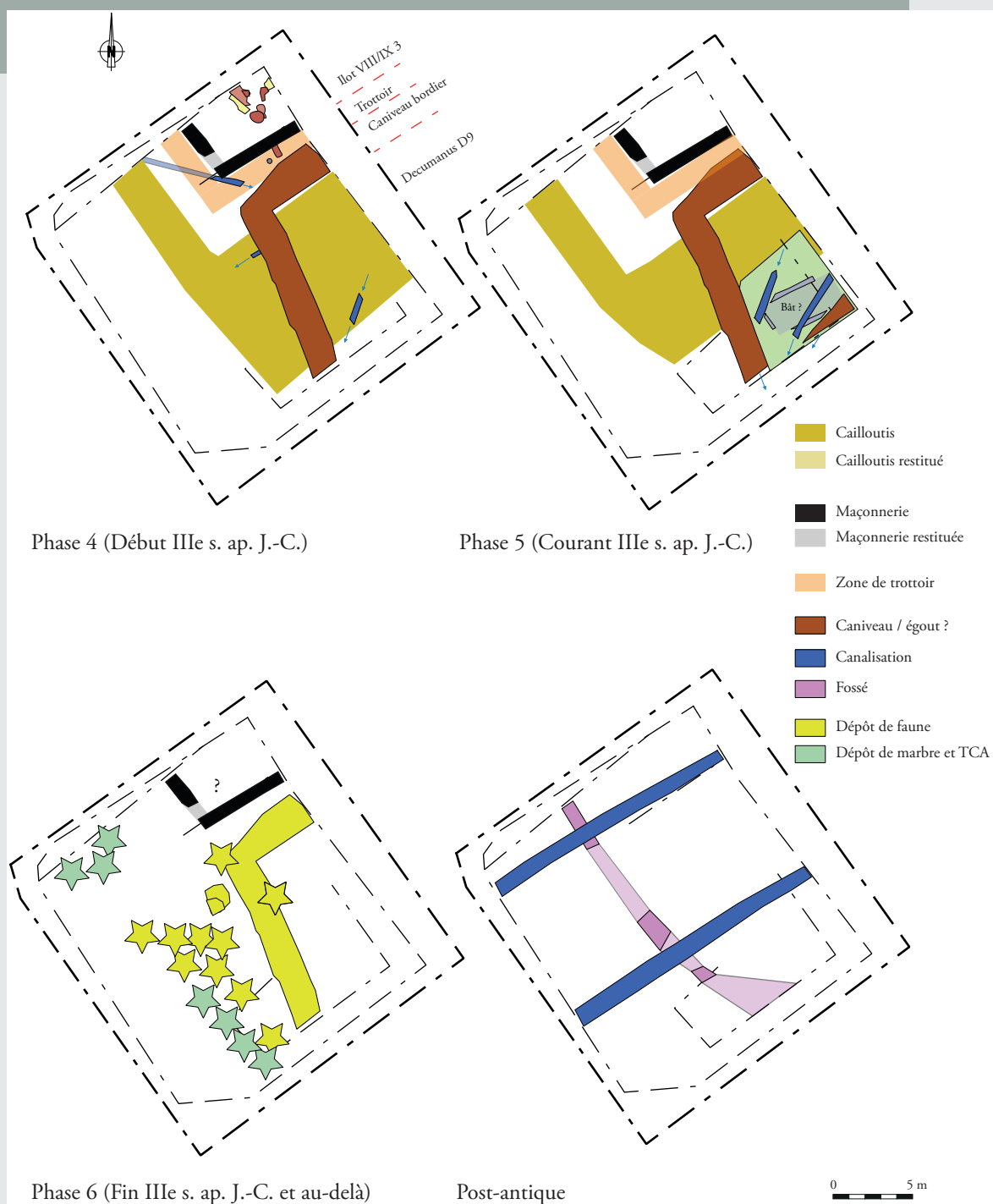
Fig. 3 Relevés planimétriques pour les phases 4 à 7 (DAO : J. Besson).
