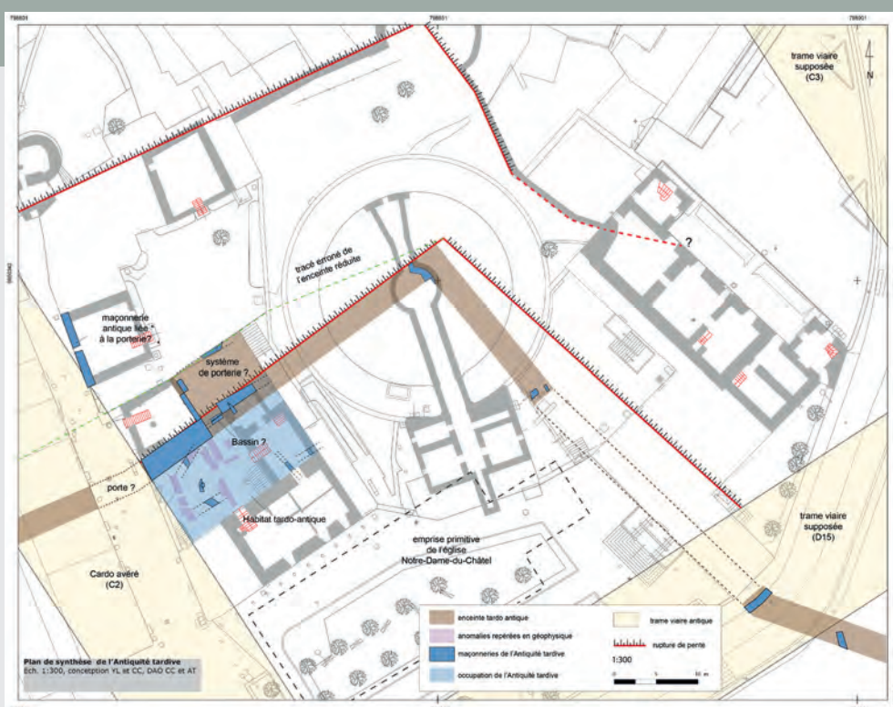
Fig. 5 Plan de synthèse des vestiges de l'Antiquité tardive (conception Y. Labaune, DAO C. Couderc et A. Tisserand).
