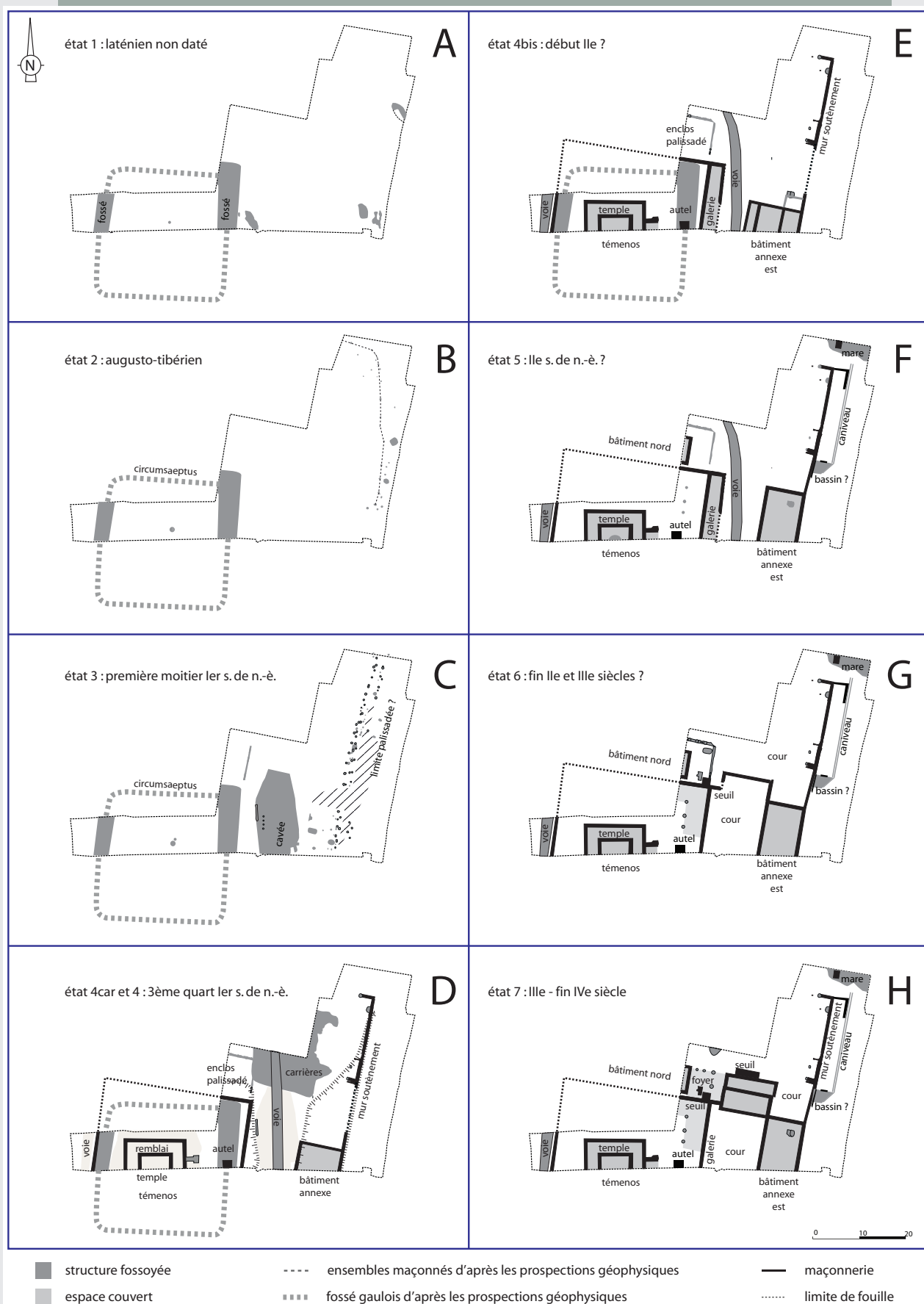
Fig. 4 Le sanctuaire de Couan à Saint-Aubin-des-Chaumes (58). Evolution du site d'après les résultats des trois premières années de fouilles (2019-2021) (DAO P. Nouvel).
