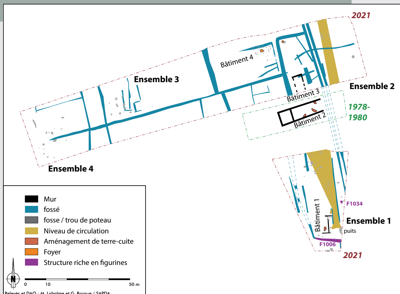
Fig. 3 Site de La Forêt , synthèse des données anciennes et de la fouille de 2021 (M. Labalme et G. Rocque – SAPDA).
